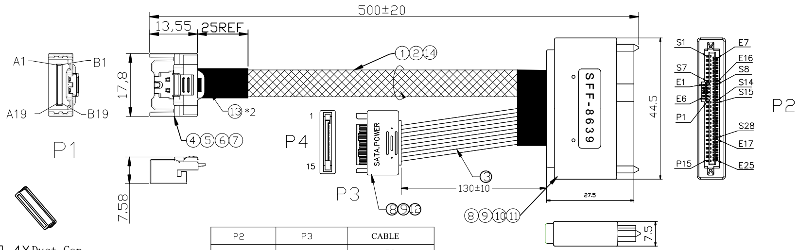
MCIO 4XDust Cap
