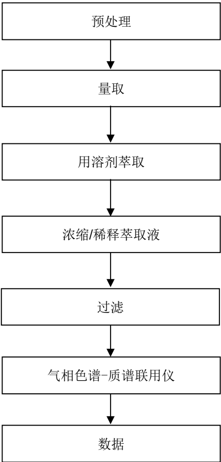
PBB(s)/PBDE(s)检测流程图
